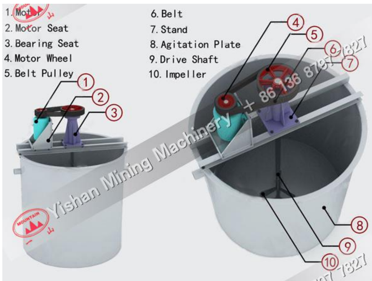
搅拌桶工作示意图
