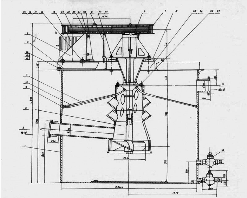
工作原理图
